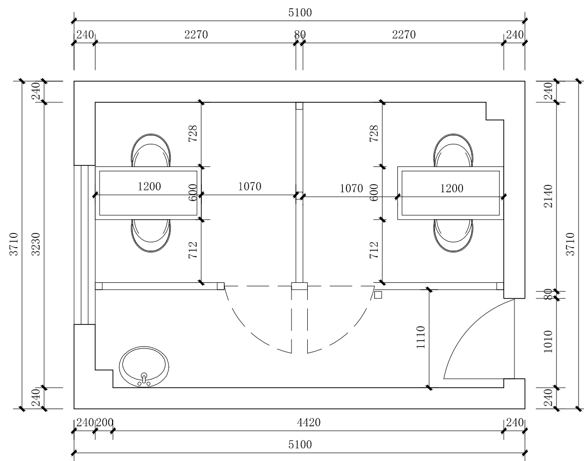
双人间平面布置图
